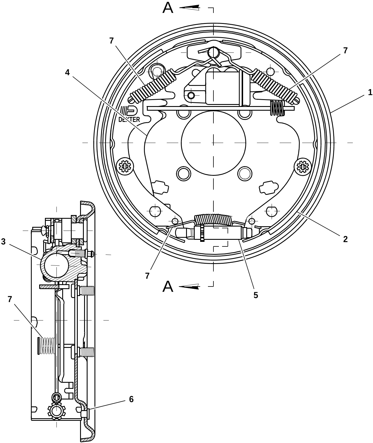
SECTION A-A
