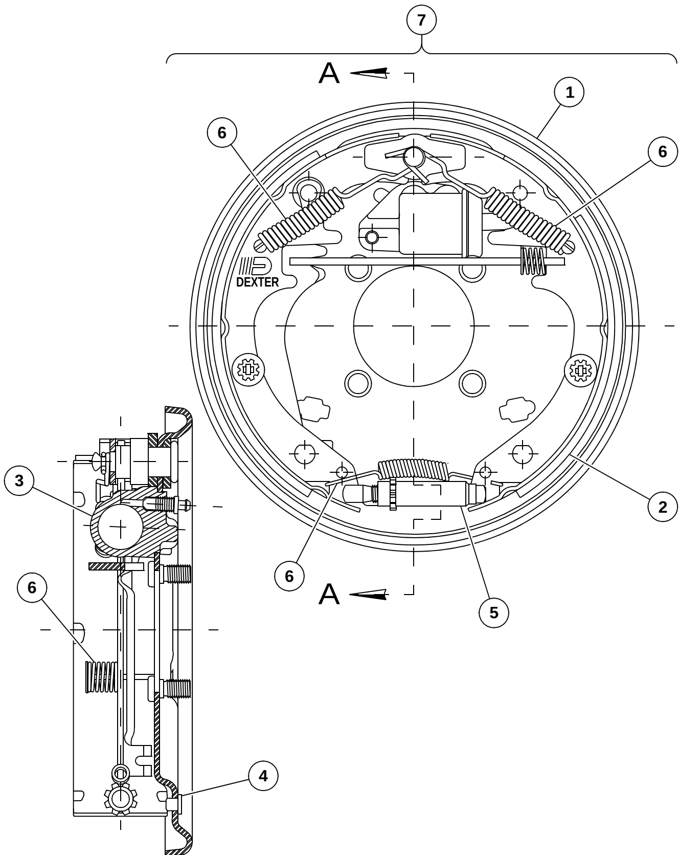
SECTION A-A
