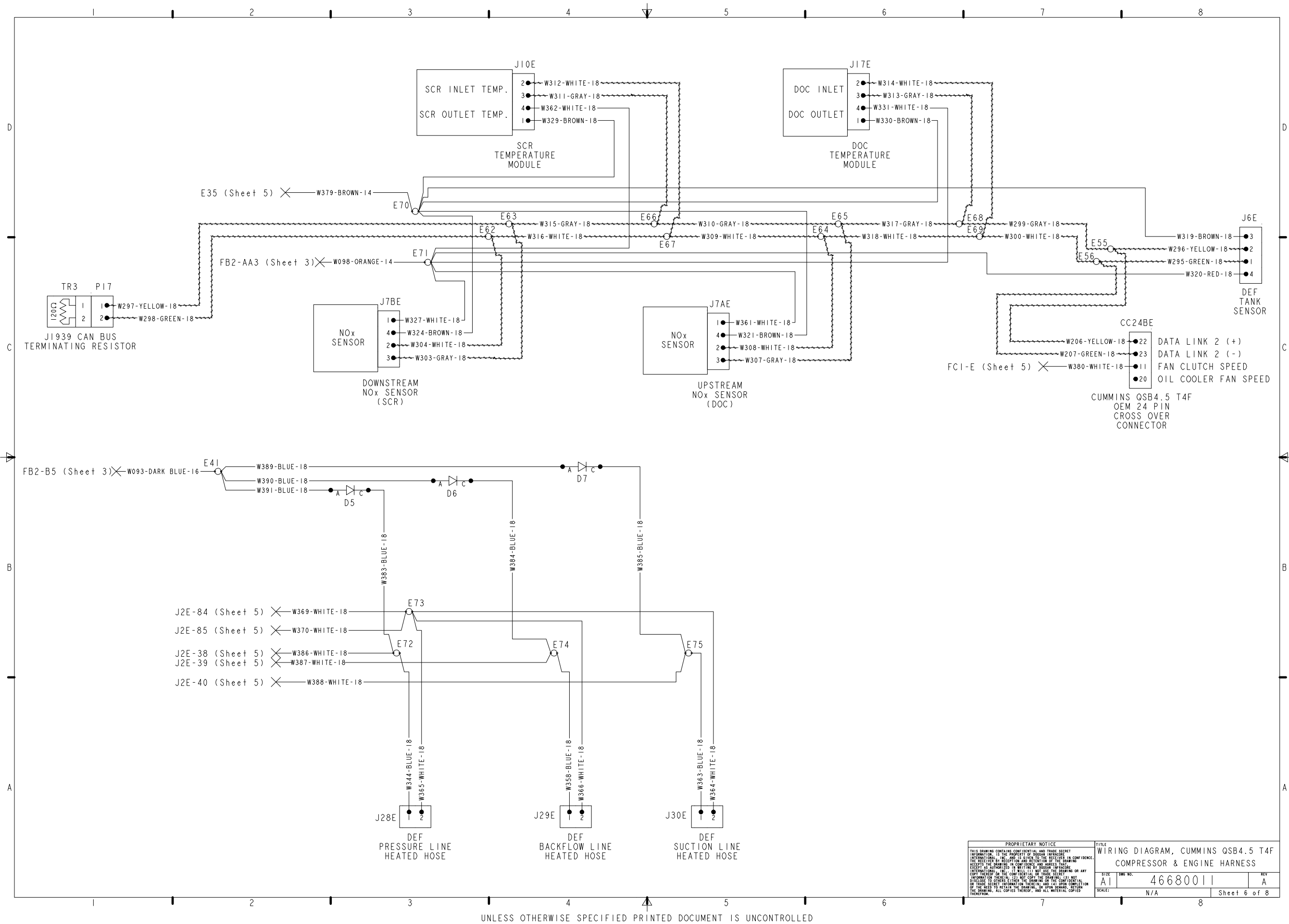
Schéma du faisceau de câblage du compresseur et du moteur 46680011 Rév.A (feuille 6 sur 8)
