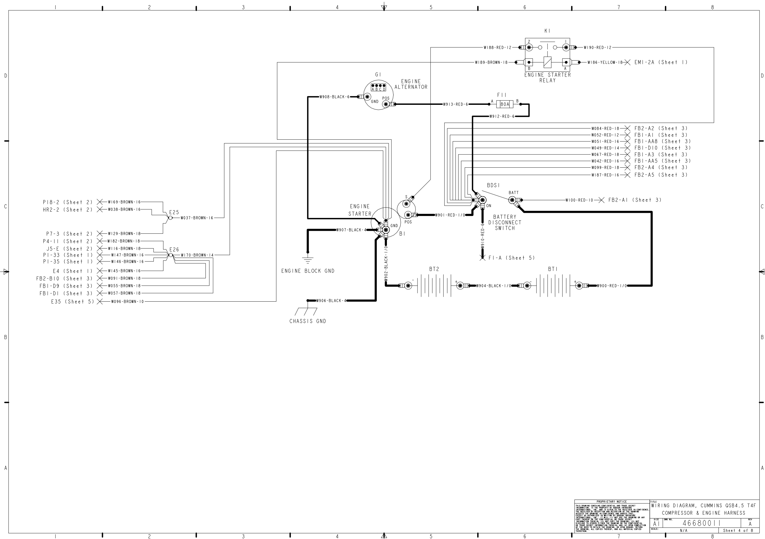
Schéma du faisceau de câblage du compresseur et du moteur 46680011 Rév.A (feuille 4 sur 8)
