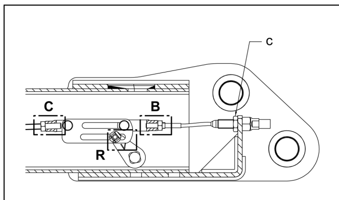
Coupe transversale montrant la position des détails B, C et R
