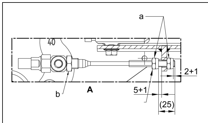
Détail A
