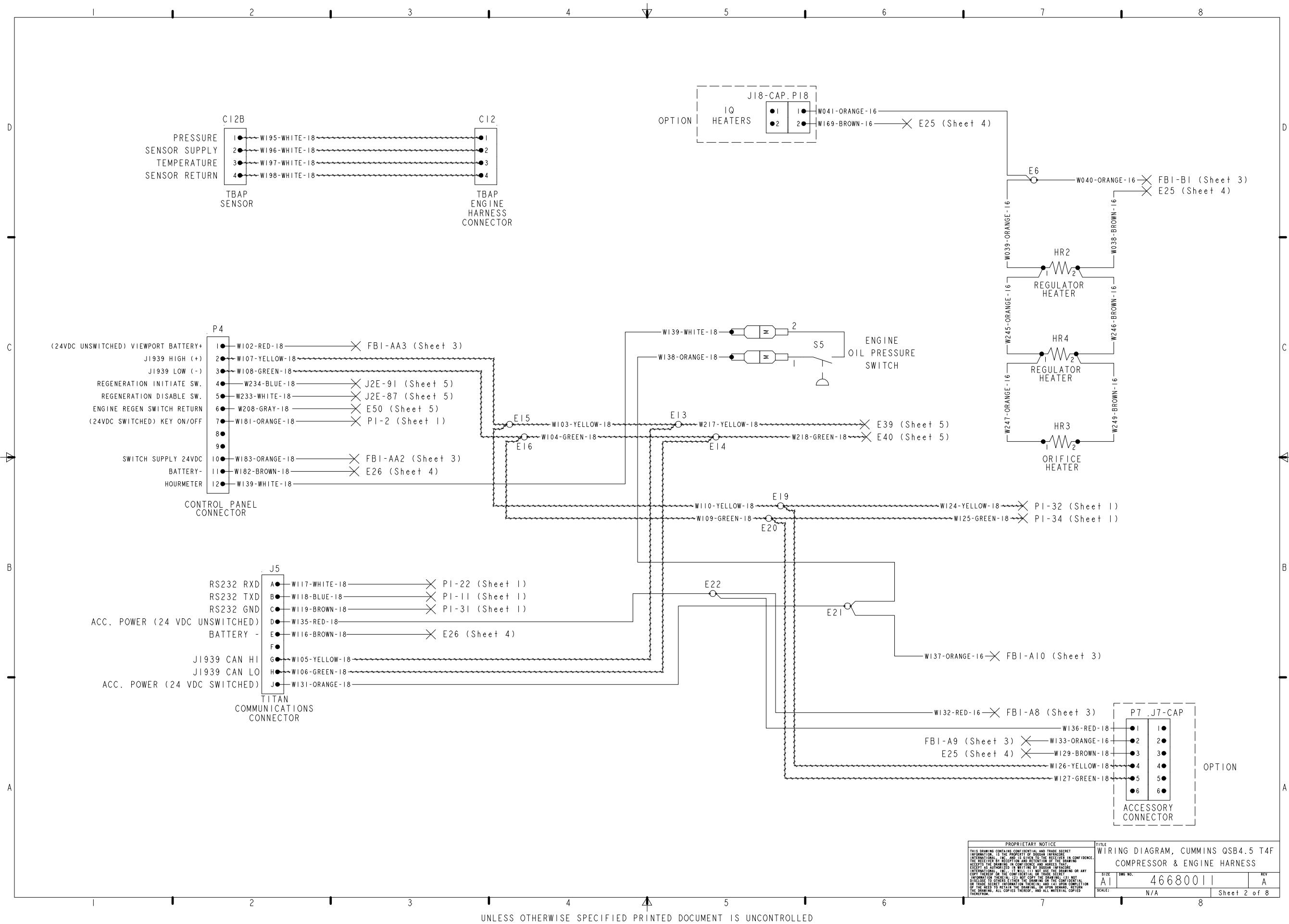
Schéma du faisceau de câblage du compresseur et du moteur 46680011 Rév.A (feuille 2 sur 8)
