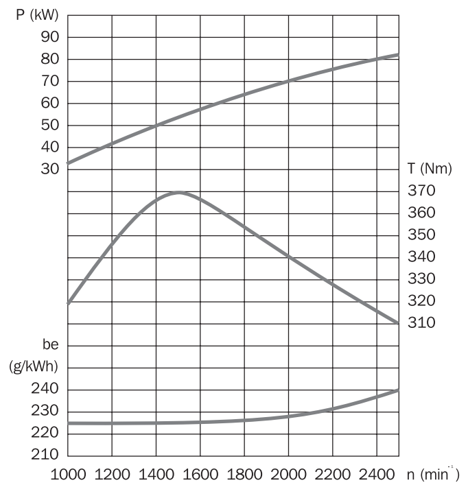
► F6L912
