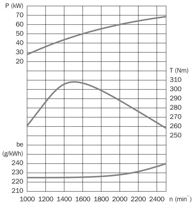
► F5L912
